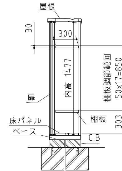
断面図
