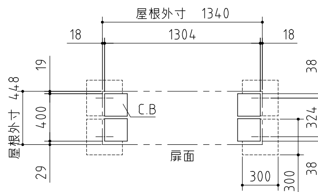
ブロック置基礎図
