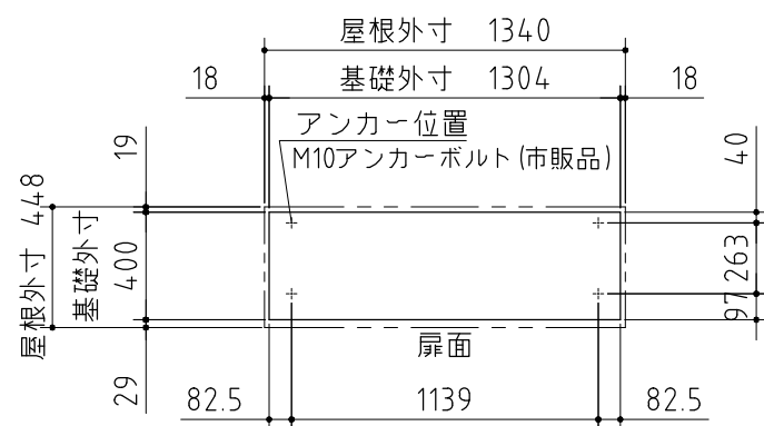
ベタ基礎図
